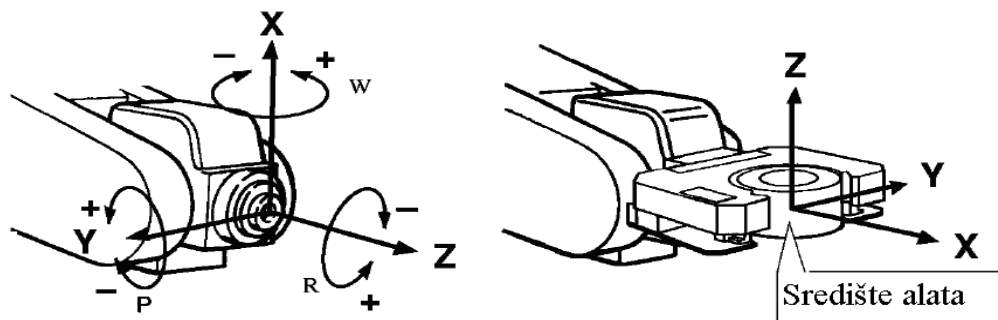
Slika 2.2. Središte alata
