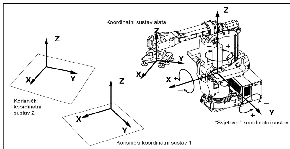
Slika 2.4. Koordinatni sustavi
