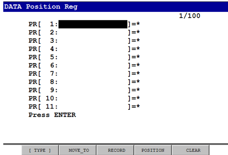
Slika 1.1. Pozicijski registri
