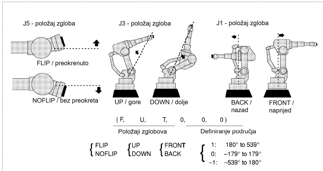
Slika 2.1. Konfiguracije robotske ruke
