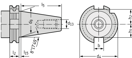
Tool adaptor (SK) DIN 69 871 part 1, form A
