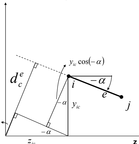
y, z osi koordinatnog sustava kroz neutralne osi poprečnog presjeka
