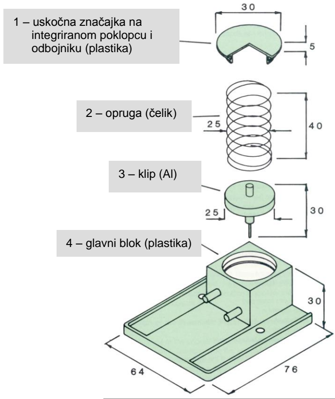
Preoblikovani pneumatski cilindar
